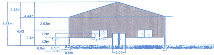
elevación frontal
